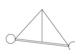
GYM SMALL P267BX214 sfera bianca /white sphere P267TX214 sfera tortora /dove sphere L 110 H 400 cm
